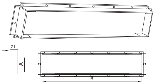
Fig.34 Entrée d'air
