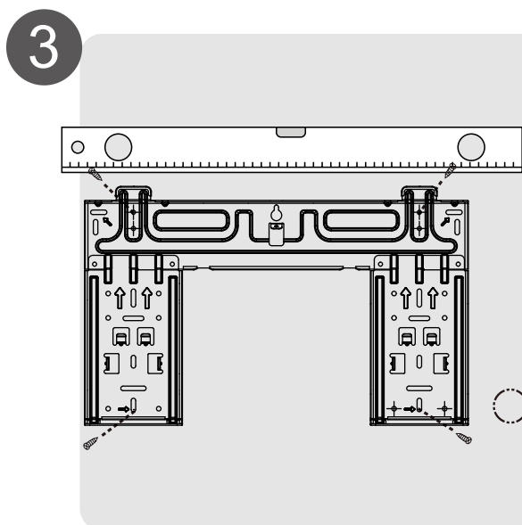
Fije la placa de montaje (Pág. 12)
