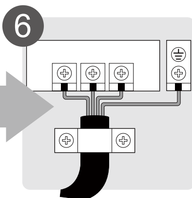
Conexión del cableado (pág. 17)
