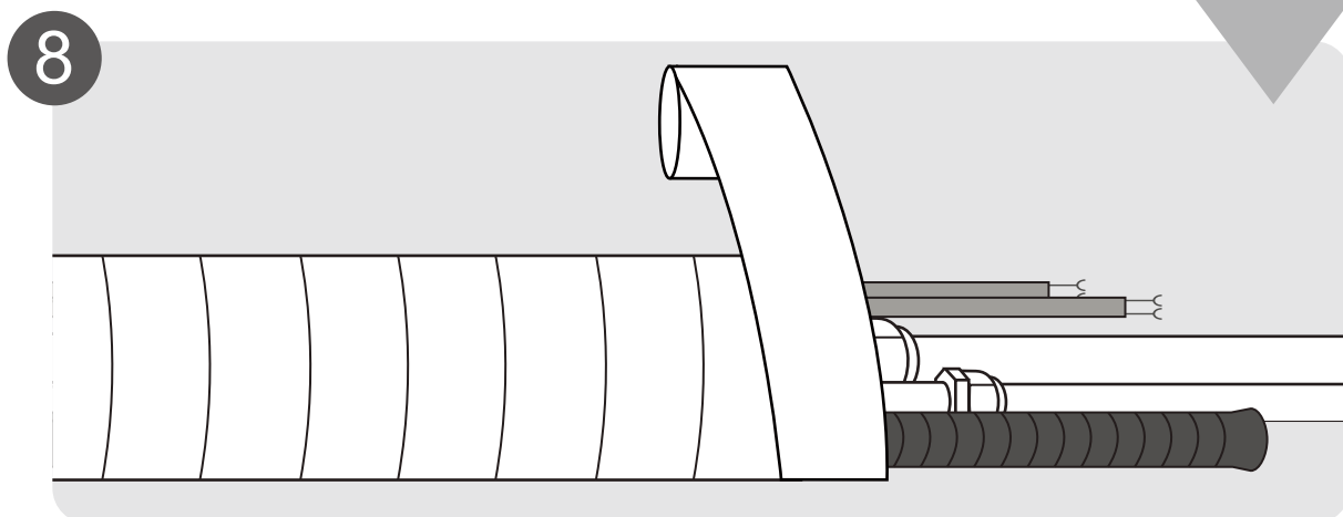
Envolver tuberías y cables (pág.18)
